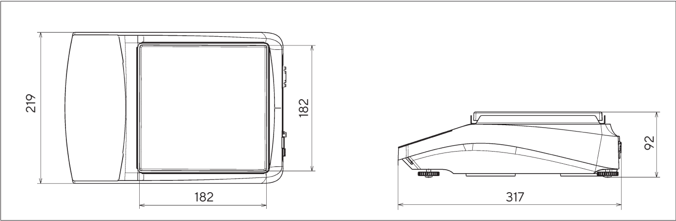
Fig. 8: Dimensiones en mm
