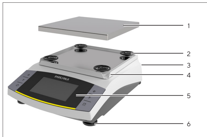
Abb.1: Präzisionswaage (Vorderansicht)
