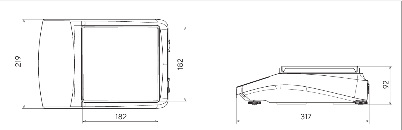
Fig. 8: Gerätemaße in mm
